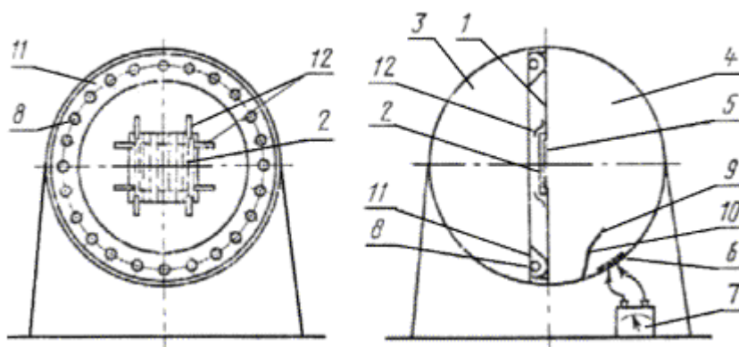
Схема диффузомера
