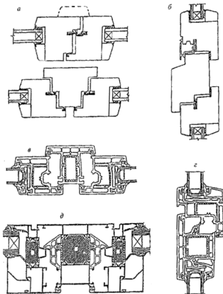
а - вертикальные безимпостный (штульповой) и импостный притворы деревянного оконного блока; б - горизонтальный импостный притвор деревянного оконного блока; в - импостный притвор оконного блока из ПВХ профилей; г - узел импостного соединения открывающейся створки и остекленной коробки; д - импостный притвор оконного блока из алюминиевого сплава
